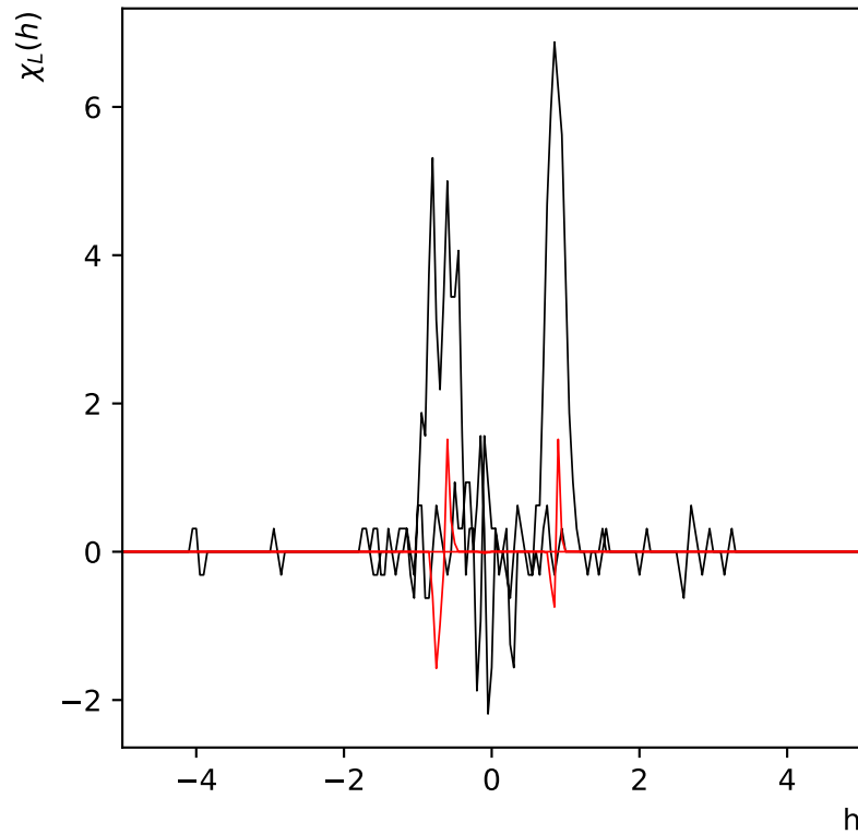
\chi_L(h) réseau de taille L=8 à T=2.0
