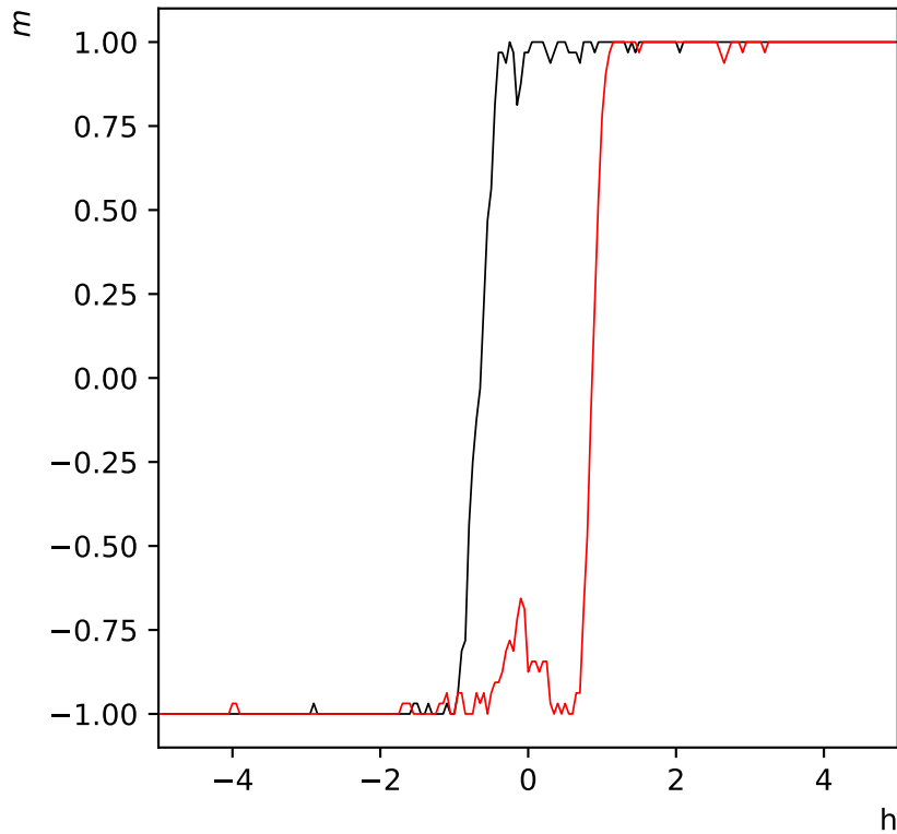
Hystérésis de l'aimantation réseau de taille L=8 - h=5 à T=2.0
